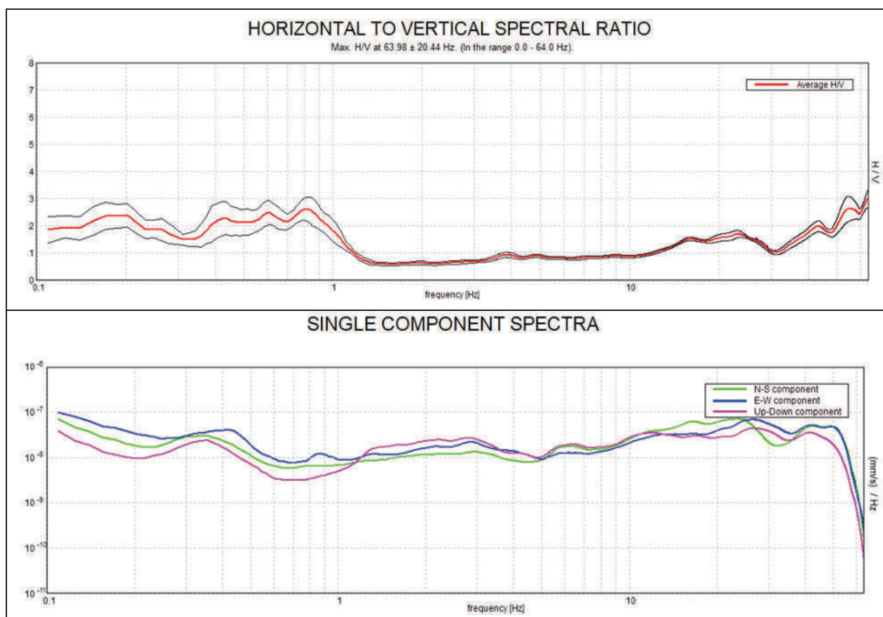
Figura 11 – Andamento degli spettri H/V e V
