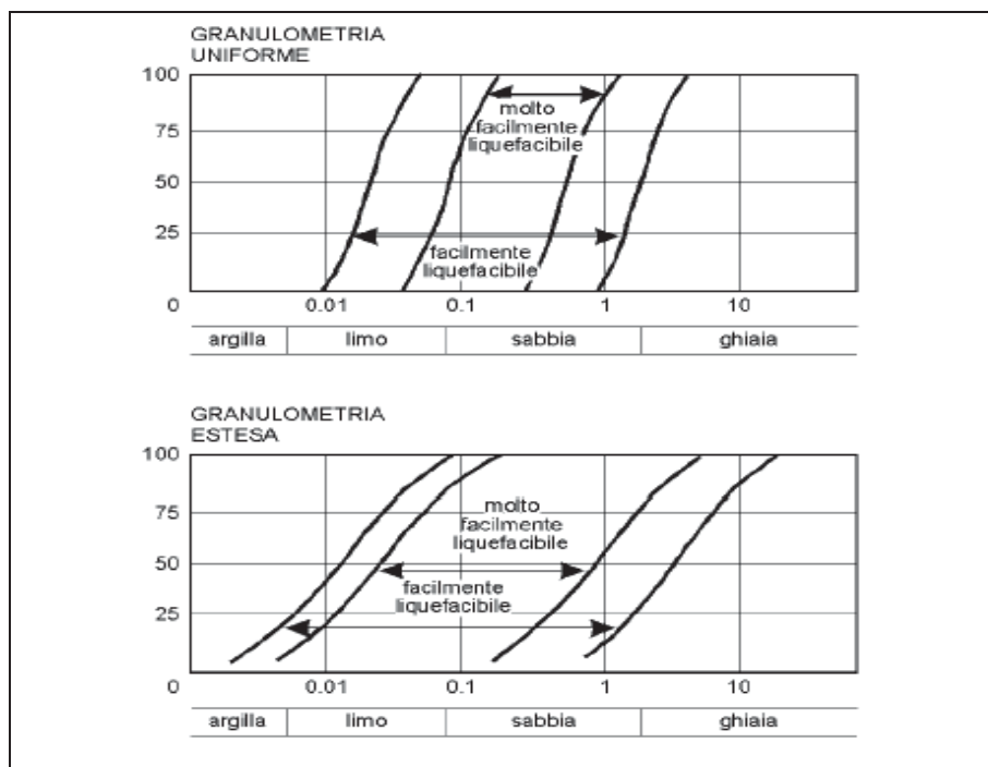
Figura 18 – Valutazione della suscettibilità alla liquefazione – fasce granulometriche critiche
