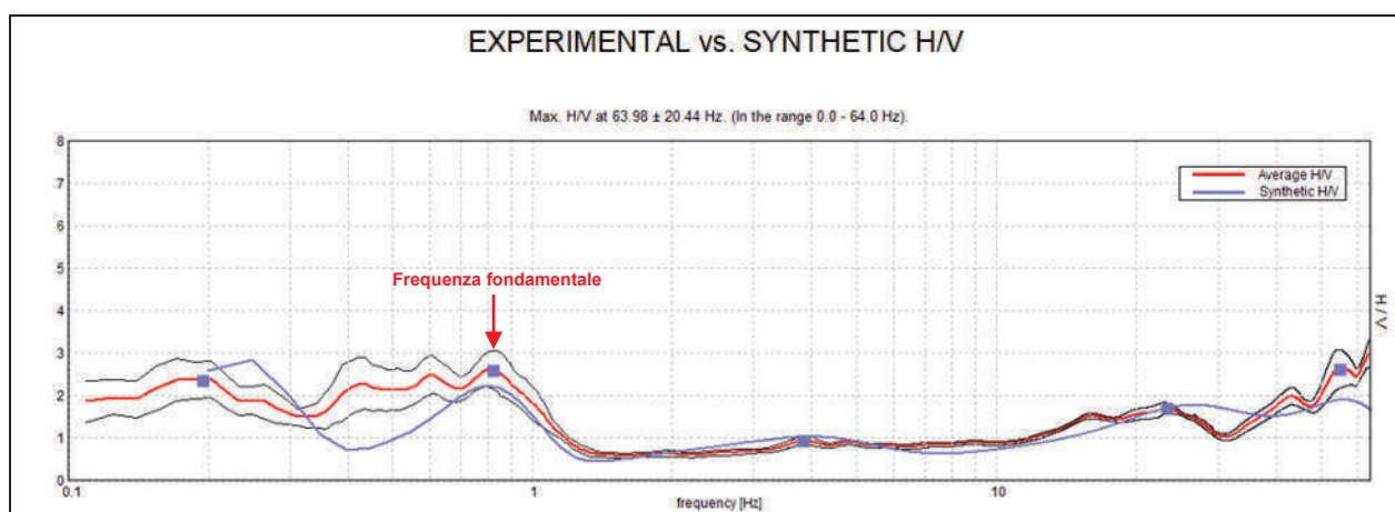
Figura 12 – Curva sintetica H/V
